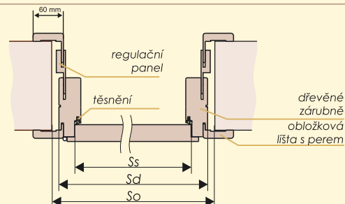
dveře s nastavitelnou zárubní Systém POL-SKONE
