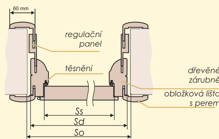
dveře s nastavitelnou zárubní Model 2000
