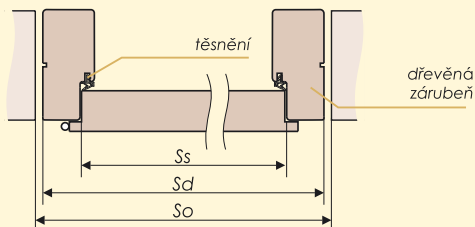
dveře s pevnou zárubní POL-SKONE
