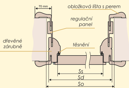
dveře s nastavitelnou zárubní MODEL RETRO
